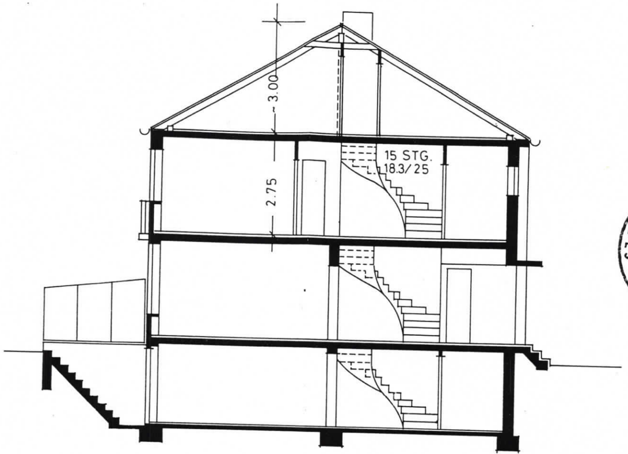
SCHNITT „A - B“
